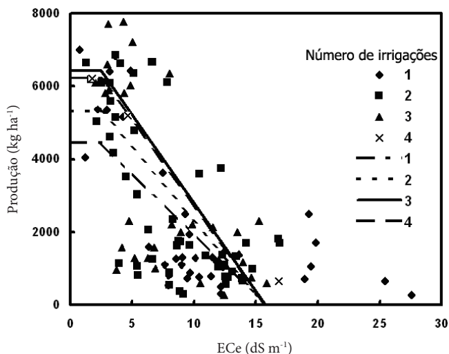
Figura 16. Efeitos da salinidade do solo a 30 cm de profundidade sobre a produção de trigo com 1, 2, 3 e 4 irrigações
