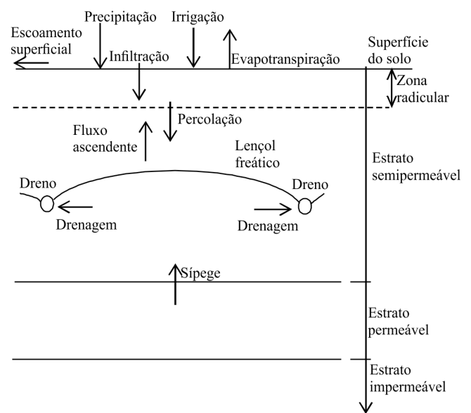
Figura 6. Representação esquemática do balanço hídrico na zona radicular e do movimento de água abaixo da zona radicular, considerando-se a drenagem artificial
