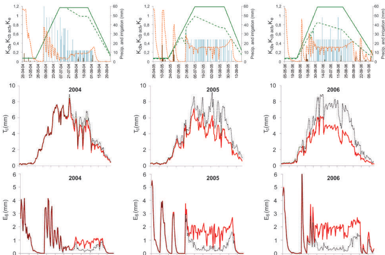
Figura 19. Valores de K_{cb\ pot} (—), K_{cb\ real} (- - - -), K_e (---), precipitação (■), e irrigação (■) da cultura do milho usando águas salinas durante as épocas de cultivo de 2004 a 2006, bem como os fluxos de transpiração ( T_c ) e evaporação do solo ( E_s ) diários potenciais (.....) e reais (—) estimados pelo modelo SIMDualKc com as correções para a salinidade
