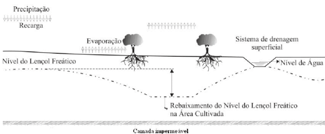
Figura 7. Utilização da biodrenagem em consórcio com o sistema de drenagem superficial, utilizado convencionalmente
