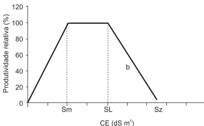
Figura 8. Representação do modelo de Sonneveld aplicado às respostas das plantas à salinidade
