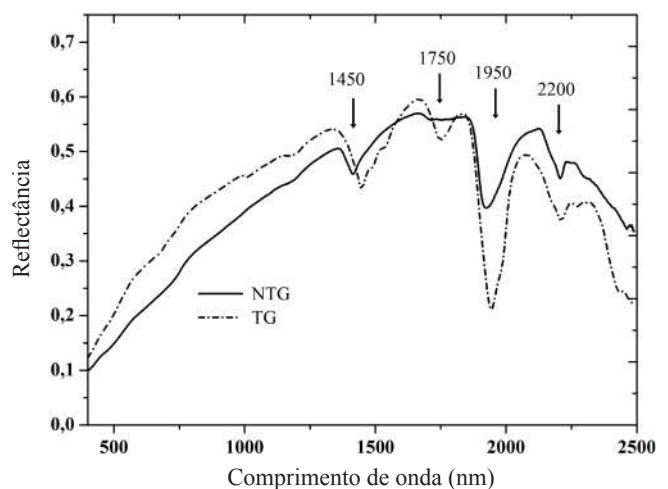
Figura 8. Espectros da CE1 de amostras de solos aluviais tratados (TG) e não tratadas (NTG) com gesso
