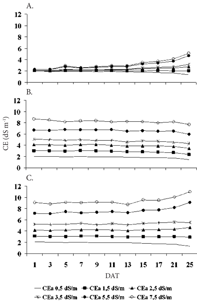
Figura 9. Variação da CE da solução nutritiva ao longo do tempo (DAT, dias após o transplantio) em função do emprego de águas salobras: apenas para reposição da evapotranspiração (A); apenas para preparo da solução nutritiva (B) e tanto para preparo da solução nutritiva quanto para reposição da evapotranspiração (C)
