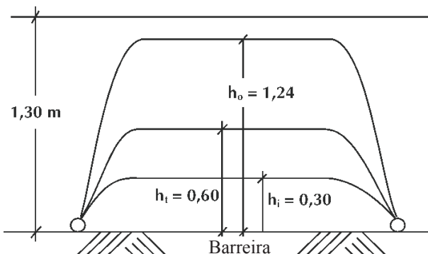
Figura 13. Esquema mostrando os parâmetros da fórmula de Boussinesq
