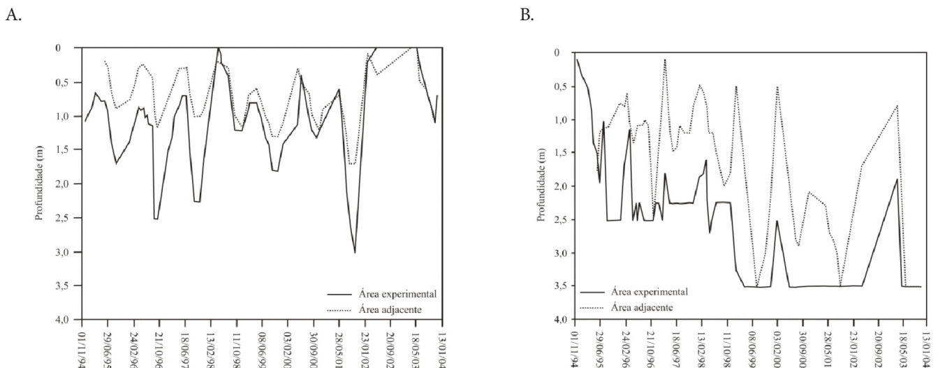
Figura 14. Comportamento do nível do lençol freático nas áreas experimentais de (A) Nahalal e (B) Genigar e em áreas nas suas adjacências no Vale Yizre'el
