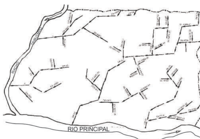
Figura 6. Desenho esquemático mostrando a nomenclatura do sistema de drenagem (NBR 14143) (ABNT, 1998a)
