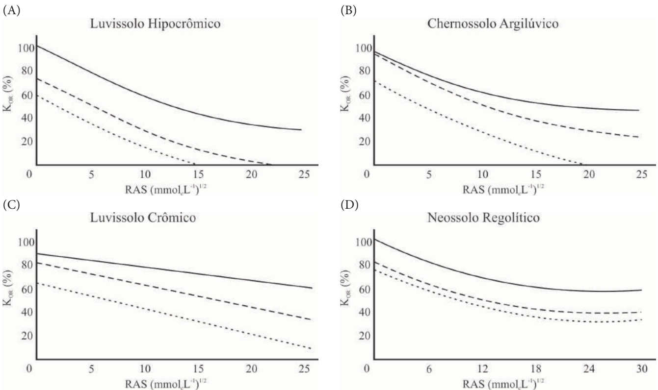
Figura 21. Condutividade hidráulica relativa ( K_{OR} ) em função da relação de adsorção de sódio (RAS) em amostras do Luvisolo Hipocrômico, Chernossolo Argilúvico, Luvisolo Crômico, e Neossolo Regolítico. Curvas determinadas por cortes nas superfícies de resposta para condutividades elétricas de 175 (.....), 500 (___) e 1.500 \mu\text{S cm}^{-1} (____), respectivamente
