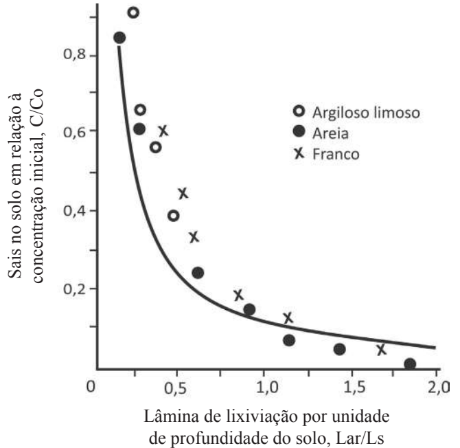
Figura 2. Lâmina de lixiviação por unidade de profundidade de solo, necessária para recuperar um solo salino por inundação intermitente
