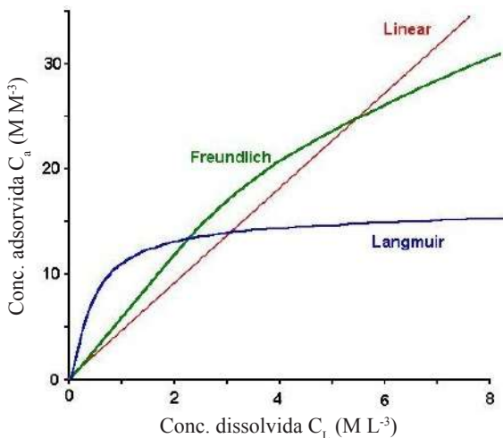
Figura 9. Formas de isotermas de adsorção
