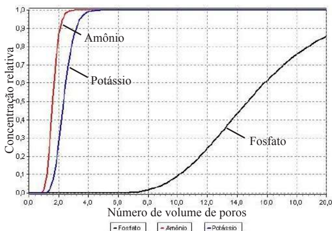
Figura 13. Curvas de efluente experimentais dos íons amônio, potássio e fosfato
