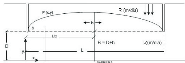
Figura 9. Desenho mostrando os parâmetros utilizados na fórmula de Hooghout
