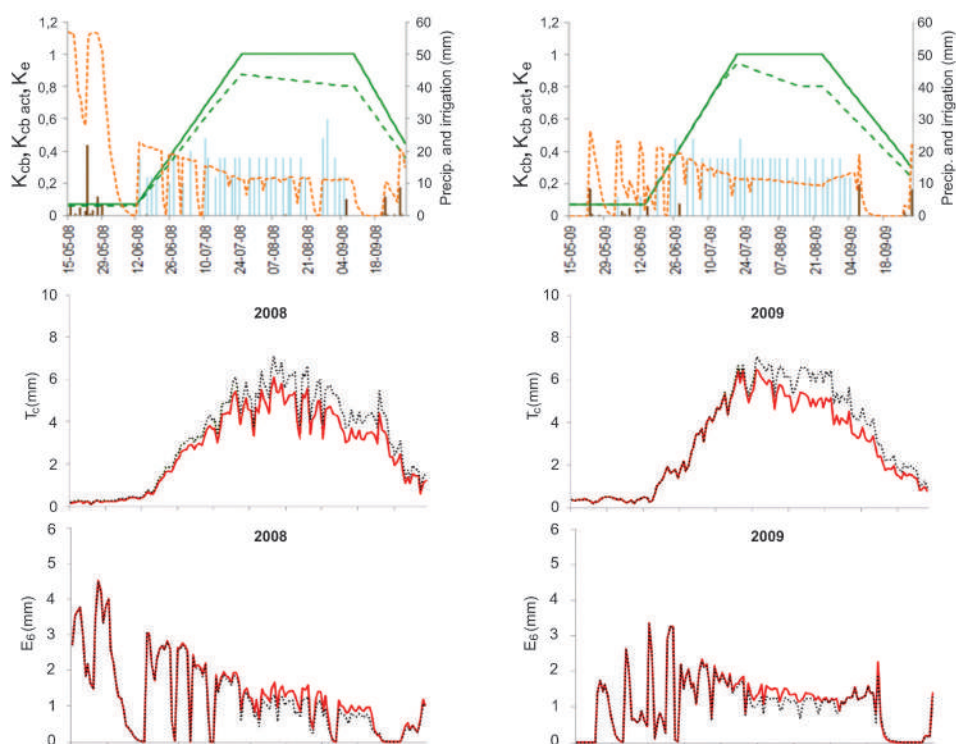
Figura 20. Valores de K_{cb\ pot} (—), K_{cb\ real} (- - - -), K_e (---), precipitação (■), e irrigação (■) da cultura do sorgo usando águas salinas durante as épocas de cultivo de 2008 a 2009, bem como os fluxos de transpiração ( T_c ) e evaporação do solo ( E_s ) diários potenciais (.....) e reais (—) estimados pelo modelo SIMDualKc com as correções para a salinidade
