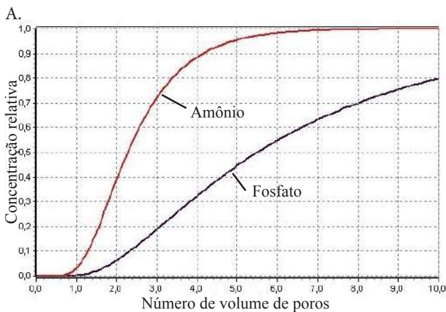
Figura 7. Curvas de efluente para um soluto com baixa e alta dispersão-difusão em um determinado solo
