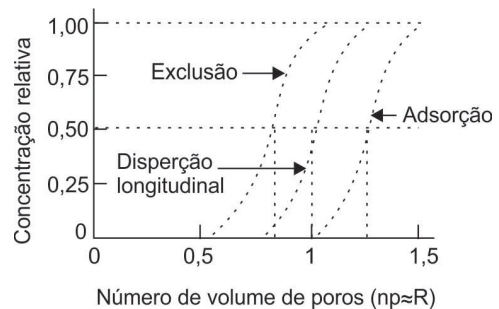
Figura 6. Curvas de efluentes para as situações em que ocorre dispersão-difusão com exclusão, dispersão-difusão apenas e dispersão-difusão com adsorção de um soluto em uma coluna de solo
