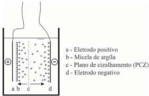
Figura 15. Separação iônica mostrando os eletrodos positivo e negativo, a micela e o plano de cisalhamento
