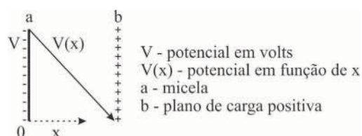
Figura 11. Geometria da teoria de Helmholtz
