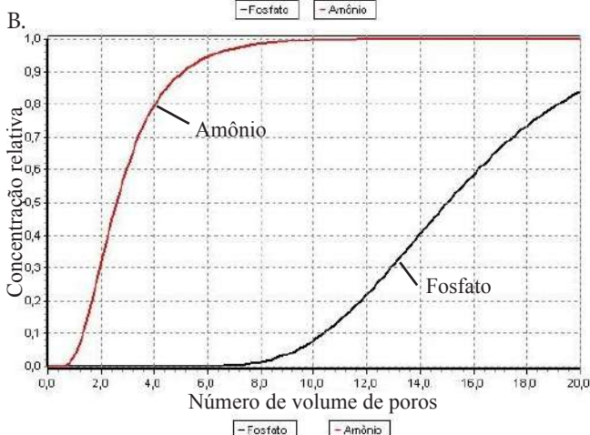
Figura 8. Curvas de efluente dos íons fosfato e amônio para um Neossolo Quartzarênico órtico (RQo) (A) e um Latossolo Vermelho distrófico (LVd) (B)
